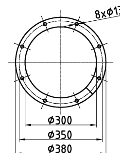
příruba P1
